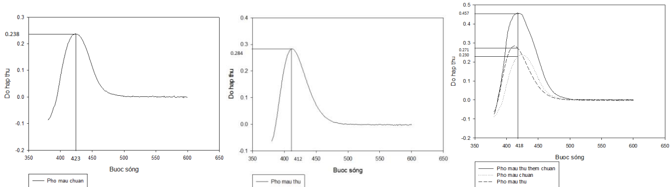
Hình 1 Phổ UV – Vis của mẫu chuẩn, mẫu thử và mẫu thử thêm chuẩn
