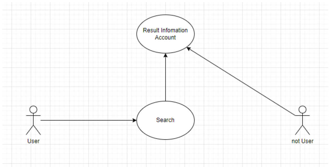
Hình 3.8: Usecase Search
