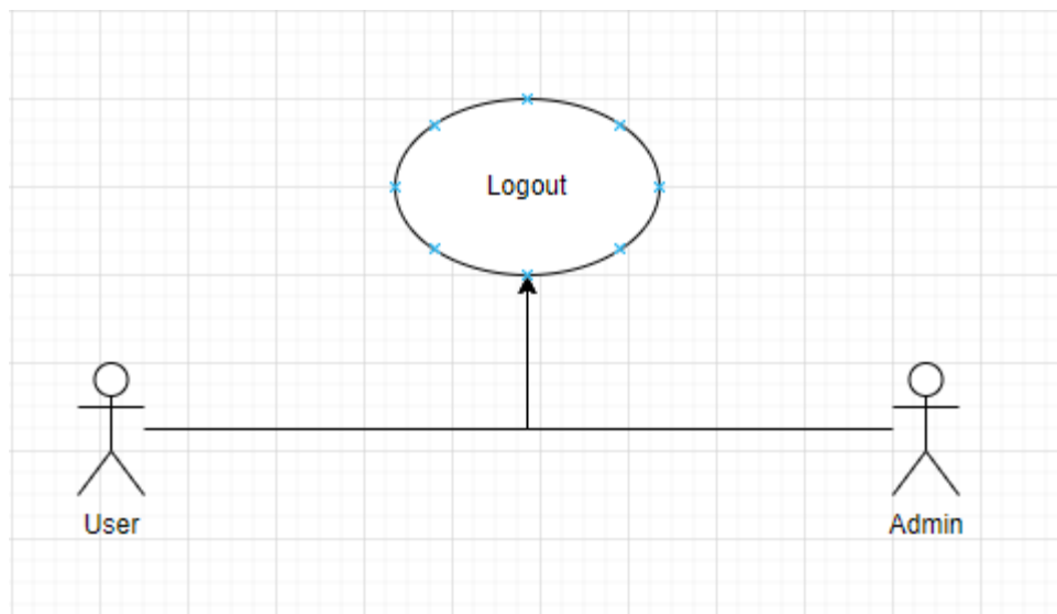
Hình 3.3: Usecase Logout
