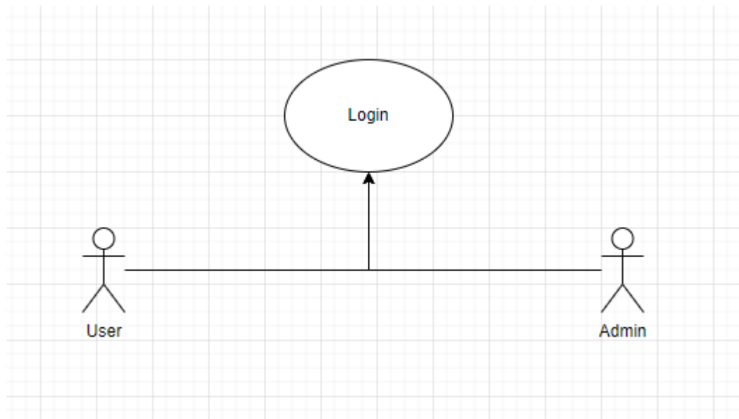
Hình 3.2: Usecase Login
