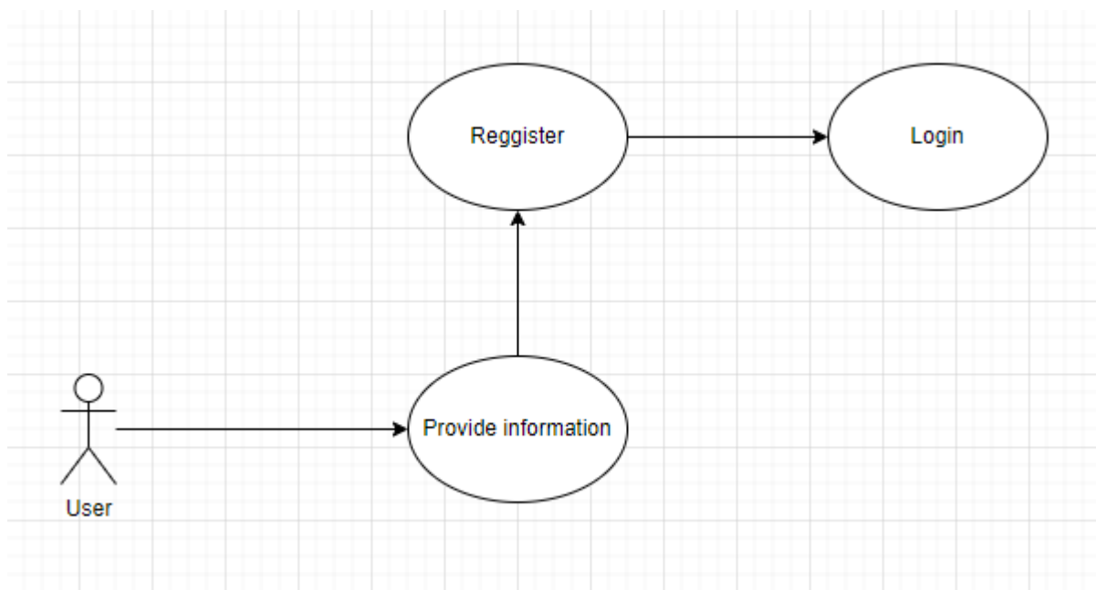
Hình 3.4: Usecase Register
